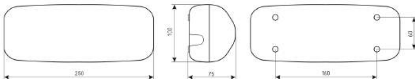
Рис. №3 Габаритный чертёж.
